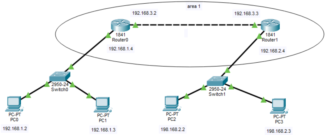
PC0
